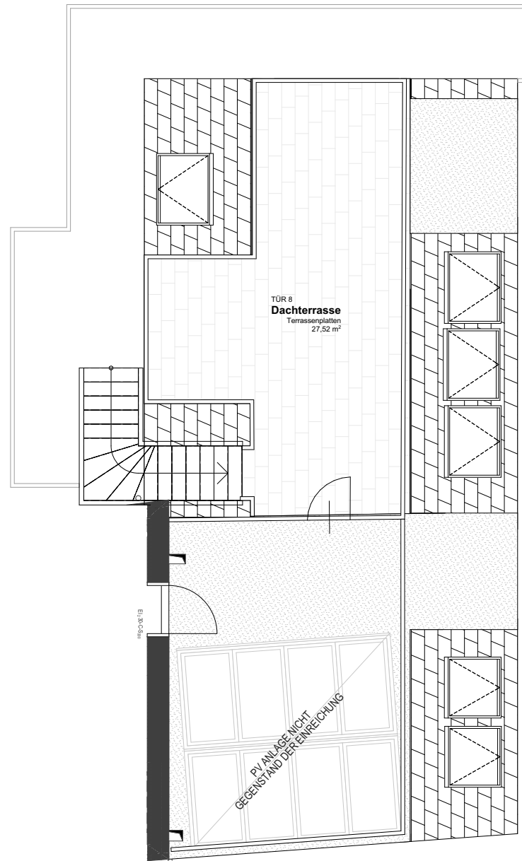
2. DACHGESCHOSS
