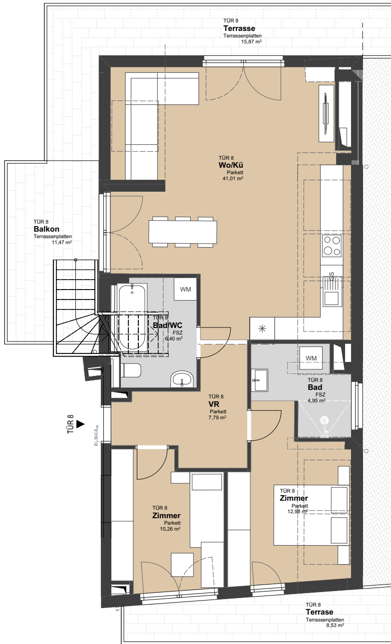
1. DACHGESCHOSS
